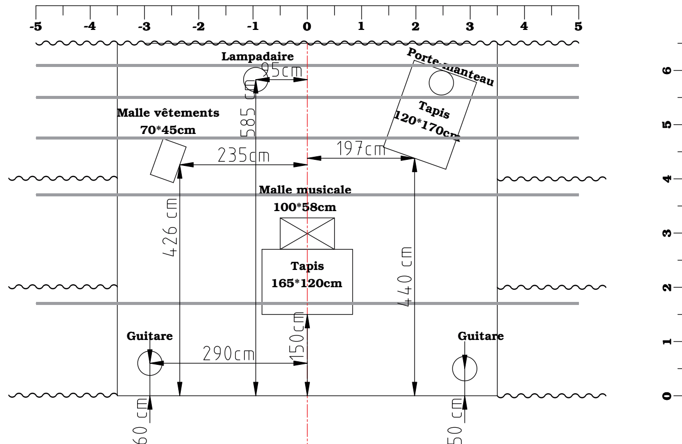
Disposition sur plateau de 7m
